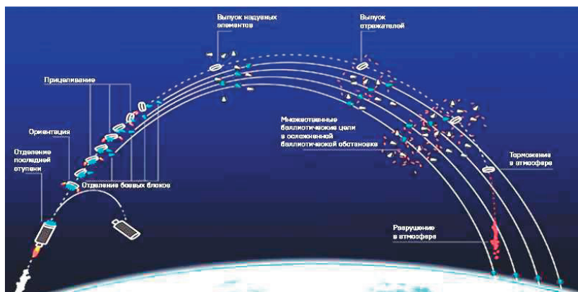
Порядок формирования сложной баллистической цели (СБЦ)
